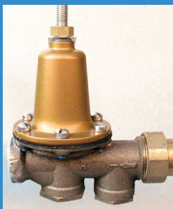
1. 压力调节器
